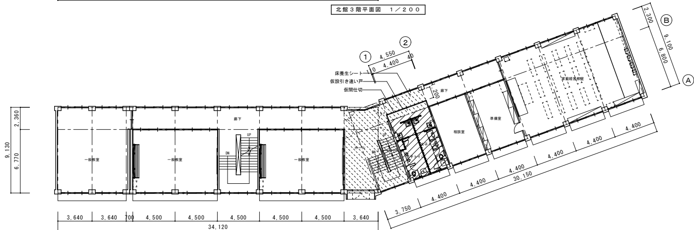
北館2階平面図 1/200
