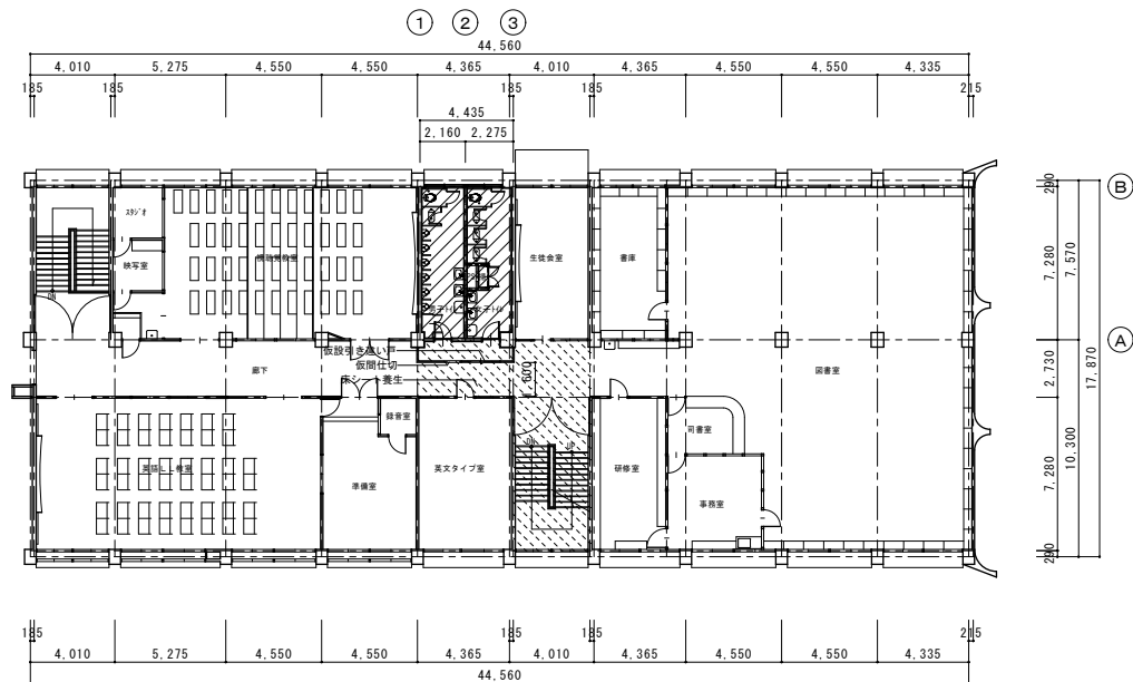
本館4階平面図 1/200
