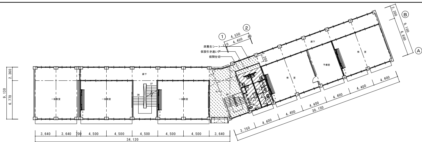
北館3階平面図 1/200
