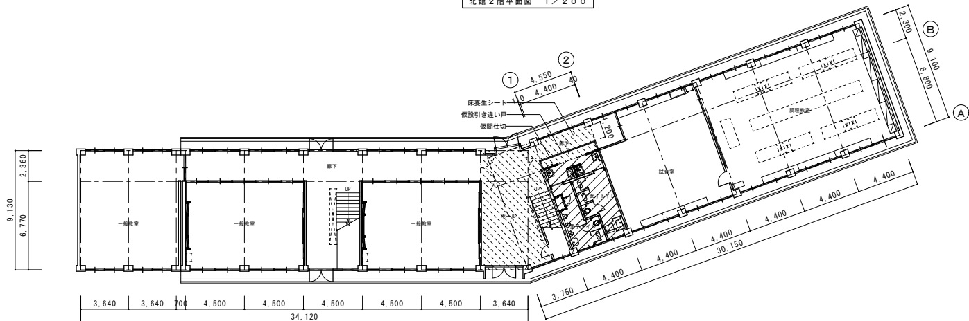
北館1階平面図 1/200
