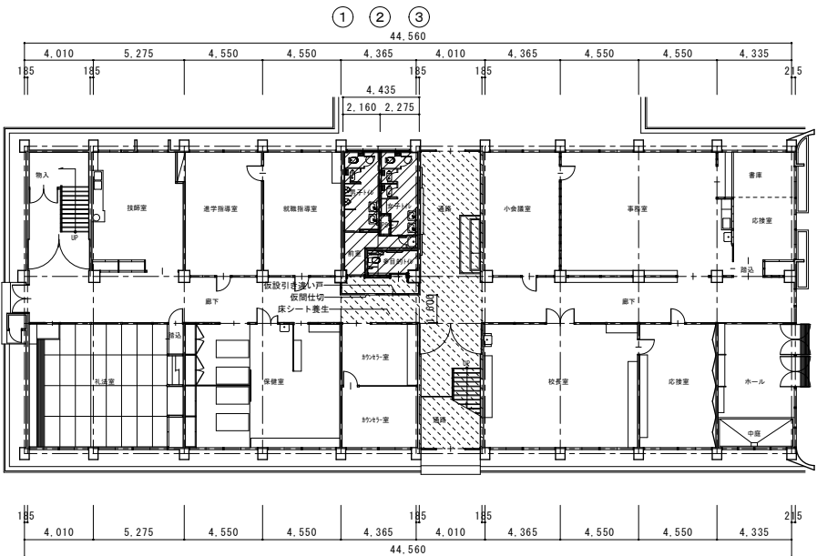
本館1階平面図 1/200
