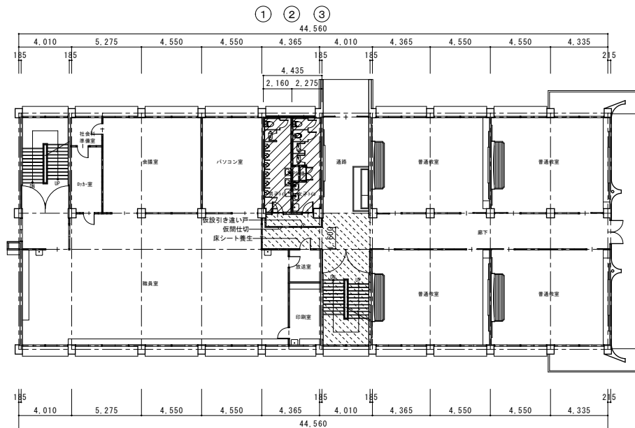
本館2階平面図 1/200
