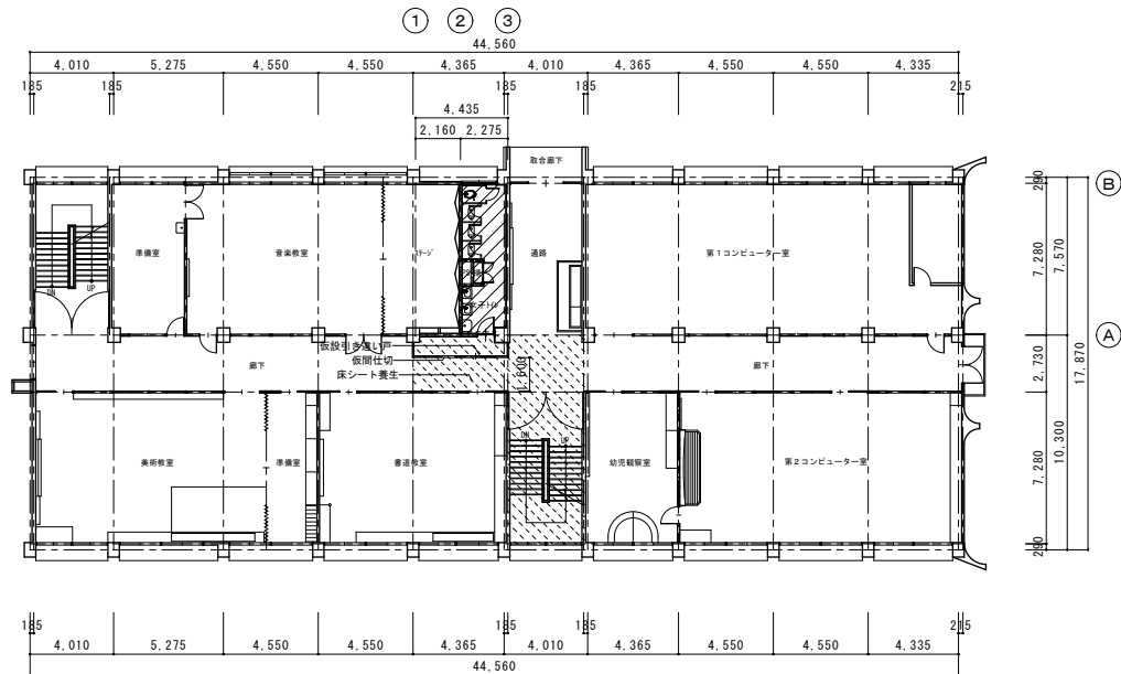
本館3階平面図 1/200
